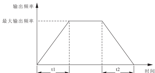
图F1-2 加速时间和减速时间示意图
