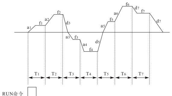
图F9-2 PLC单循环示意图
