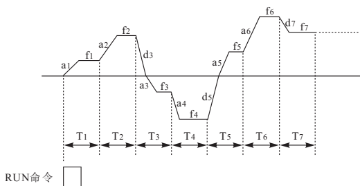
图F9-4 简易PLC运行示意图
