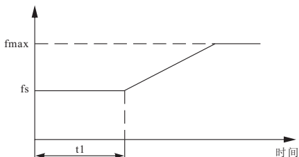
图F2-1 起动频率示意图
