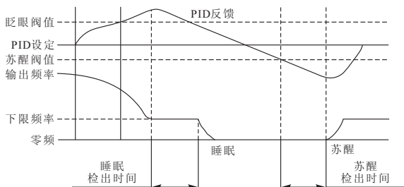
图F8-4 睡眠与苏醒功能示意图
