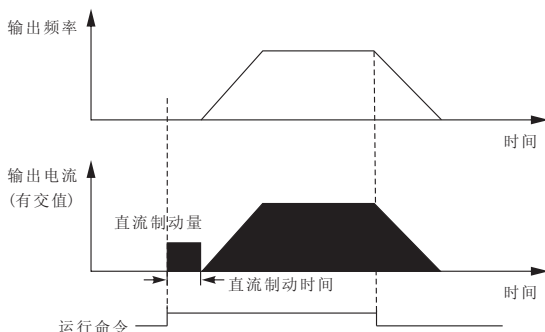
图F2-2 起动直流制动示意图
