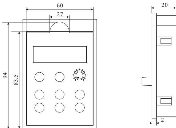
通用型操作面板外形尺寸图
