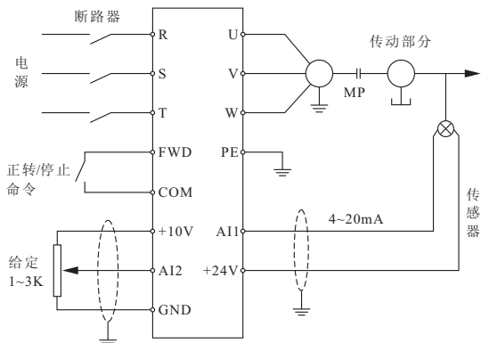
图F8-1 模拟反馈控制系统示意图
