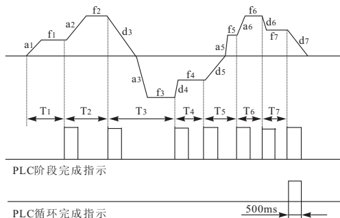
图F9-1 简易PLC运行示意图
