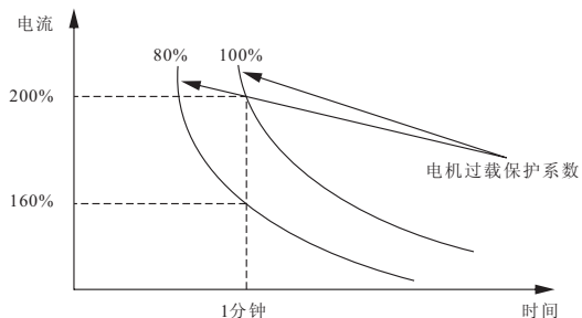
图FA-1 电机过载保护曲线示意图
