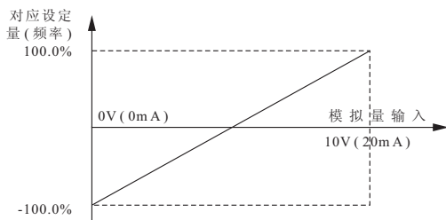
图F7-1 输入模拟量与频率关系对应示意图
