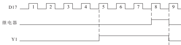
图F6-7 计数器复位设定和计数器检测设定示意图
