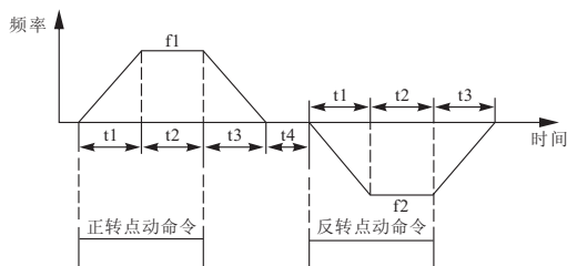
F2-4 点动运行图
