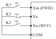
图F6-3 三线式控制模式1示意图
