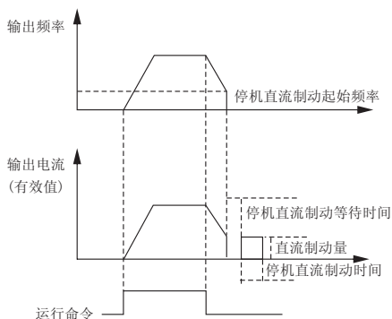
图F2-3 停机直流制动示意图
