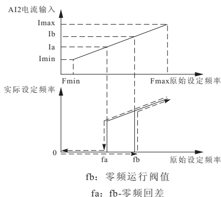
图F7-2 零频功能示意图
