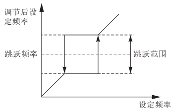
F2-5 跳跃频率设定图
