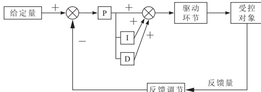
图F8-2 PID调节示意图
