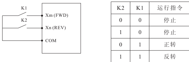
图F6-2 二线式控制模式2示意图
