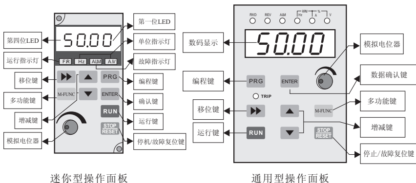
图1 LED操作面板示意图
