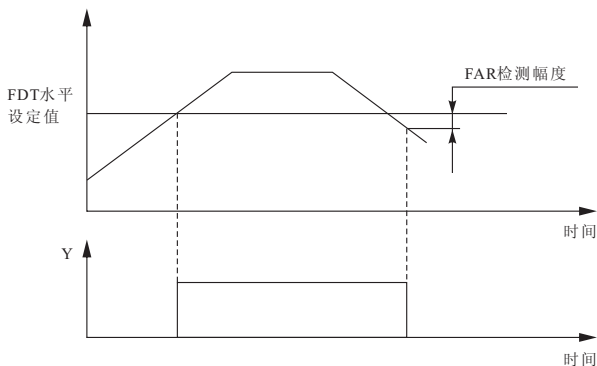
图F6-6 频率水平检测示意图
