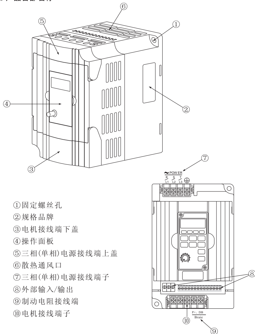
0.75~2.2KW 外形示意图
