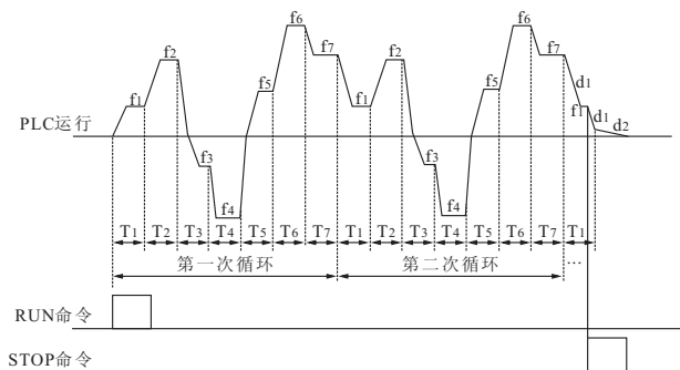
图F9-3 PLC连续示意图
