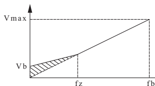
图F3-2 转矩提升示意图
