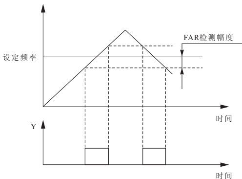
图F6-5 频率到达示意图
