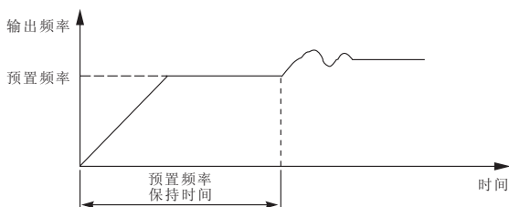
图F8-3 闭环预置频率运行示意图
