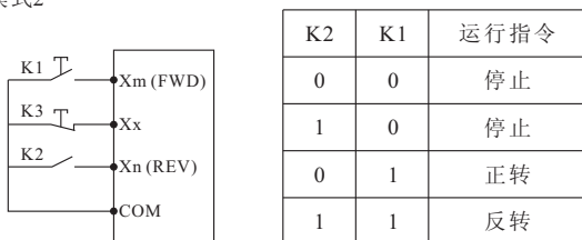
图F6-4 三线式控制模式2示意图
