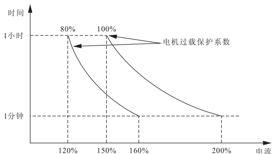
图FA-2 电机过载保护系数设定示意图
