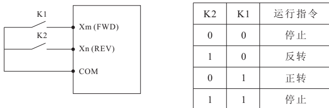
图F6-1 二线式控制模式1示意图
