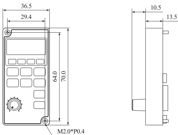
迷你型操作面板外形尺寸图
