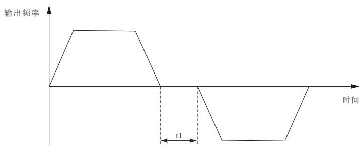
图F2-6 正反转死区时间示意图
