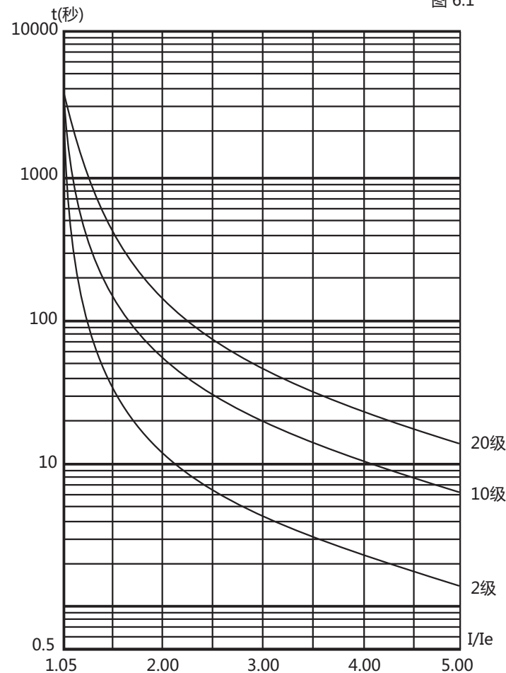
电机热保护脱扣时间曲线(热状态)
